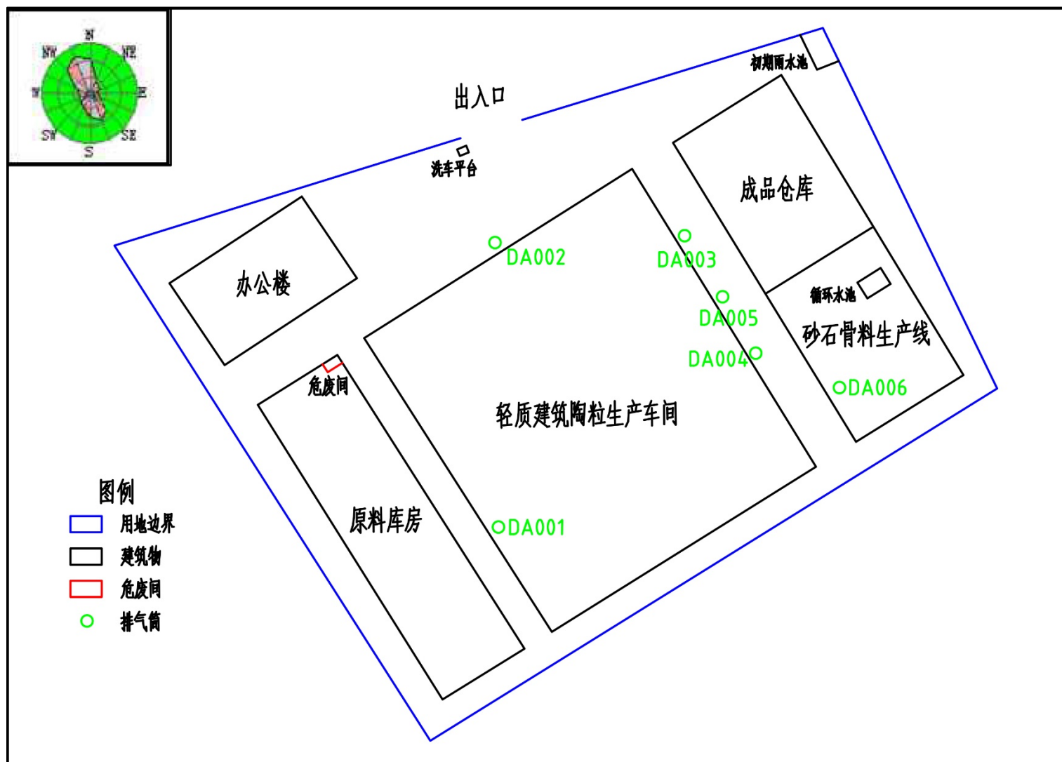
附图3 本项目平面布置图
