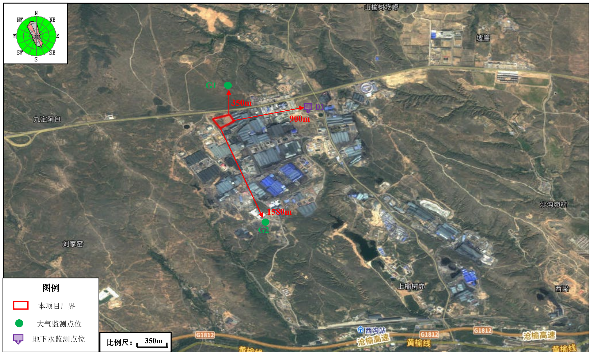
附图4 本项目监测点位图
