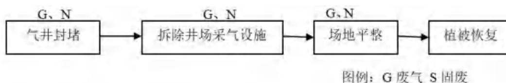
图四 闭井期工艺流程及排污节点图
