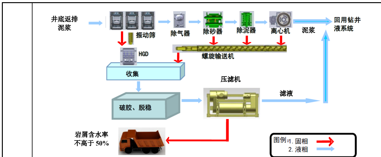
图2-4 泥浆不落地系统工艺流程简图
