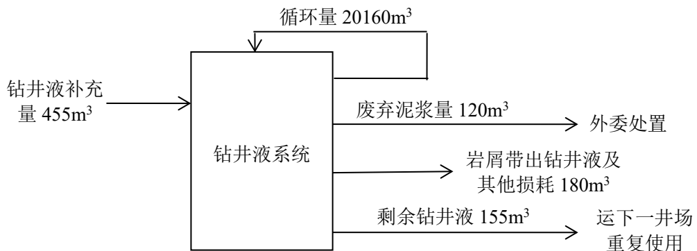
图2-2 钻井液循环量示意图
