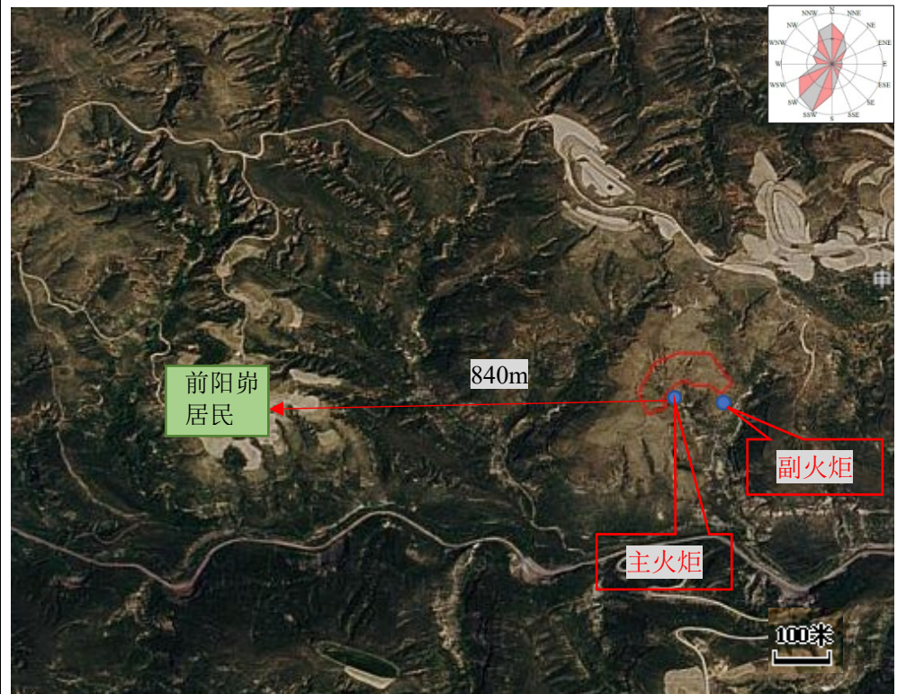
图1-2 项目火炬与最近环境保护目标位置关系图
