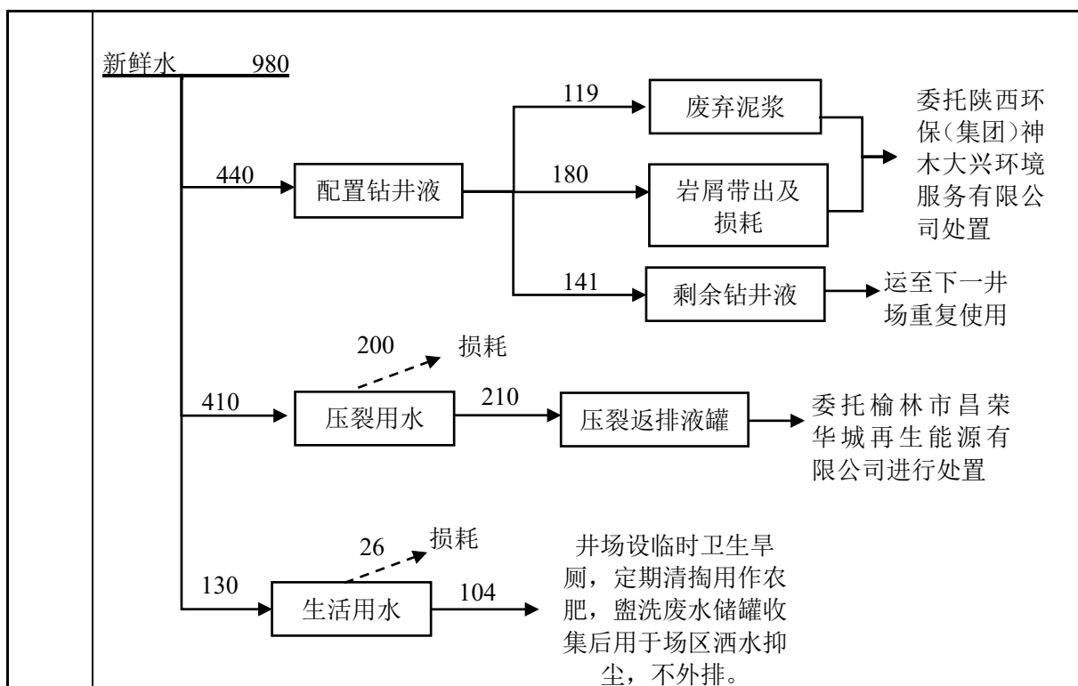
图2-3 项目水平衡图 单位：m 3
