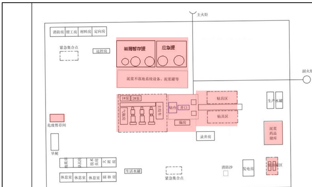
图4-1 井场防渗分区图
