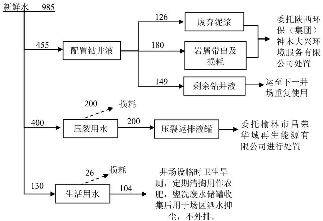
图2-3 项目水平衡图 单位：m 3
