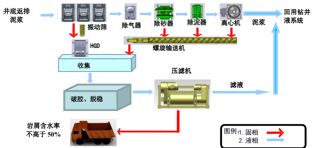
图2-4 泥浆不落地系统工艺流程简图
