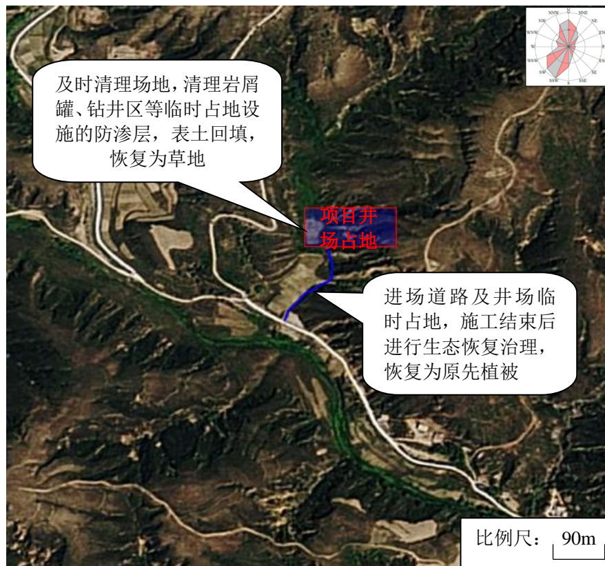
图 5-1 典型生态环境保护措施平面布置示意图
