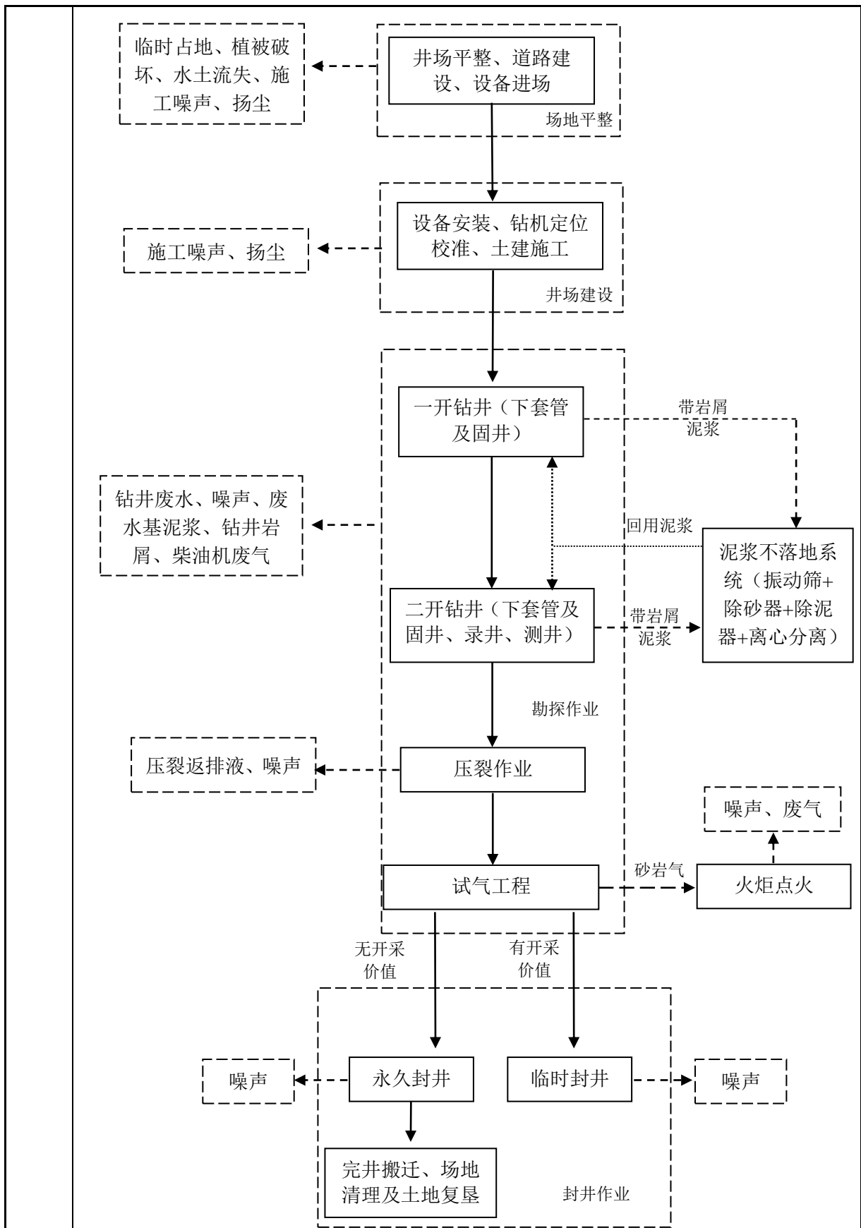
图 2-4 项目施工期工艺流程及产排污环节图
