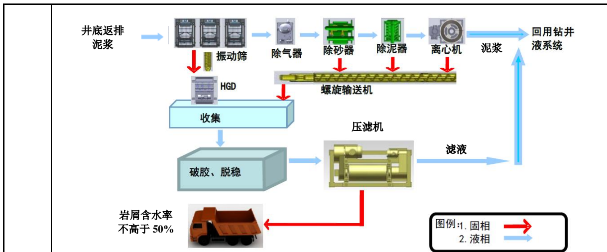
图 2-3 泥浆不落地系统工艺流程简图
