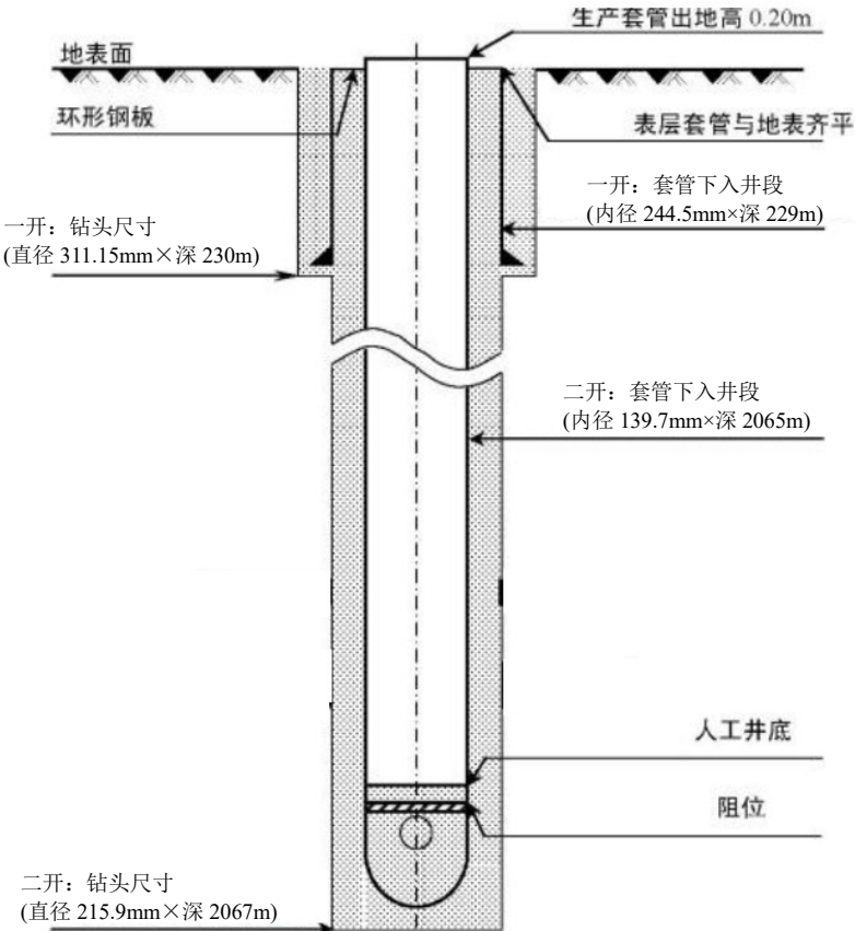
图 2-1 井身结构图
