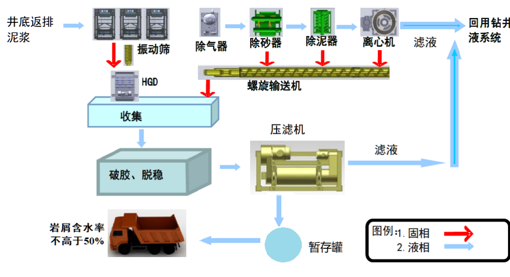
图 2-3 泥浆不落地系统工艺流程简图
