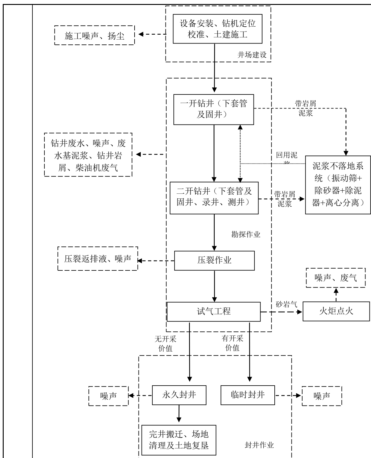
图 2-4 项目施工期工艺流程及产排污环节图
