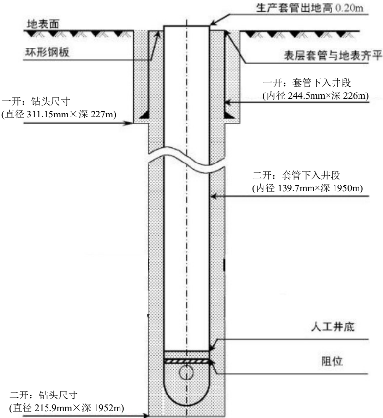
图 2-1 井身结构图
