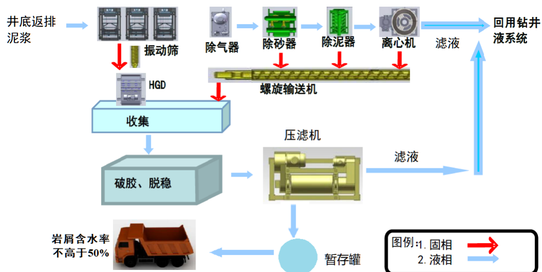
图 2-3 泥浆不落地系统工艺流程简图
