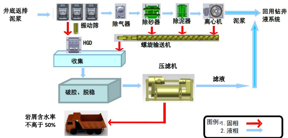
图 2-2 泥浆不落地系统工艺流程简图
