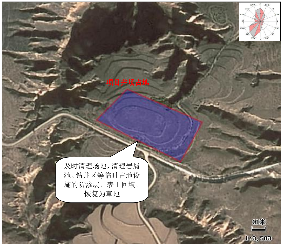
图 5-1 典型生态环境保护措施平面布置示意图
