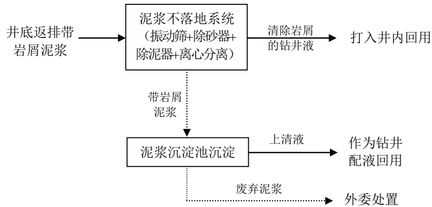
图 5 泥浆循环利用工艺流程简图
