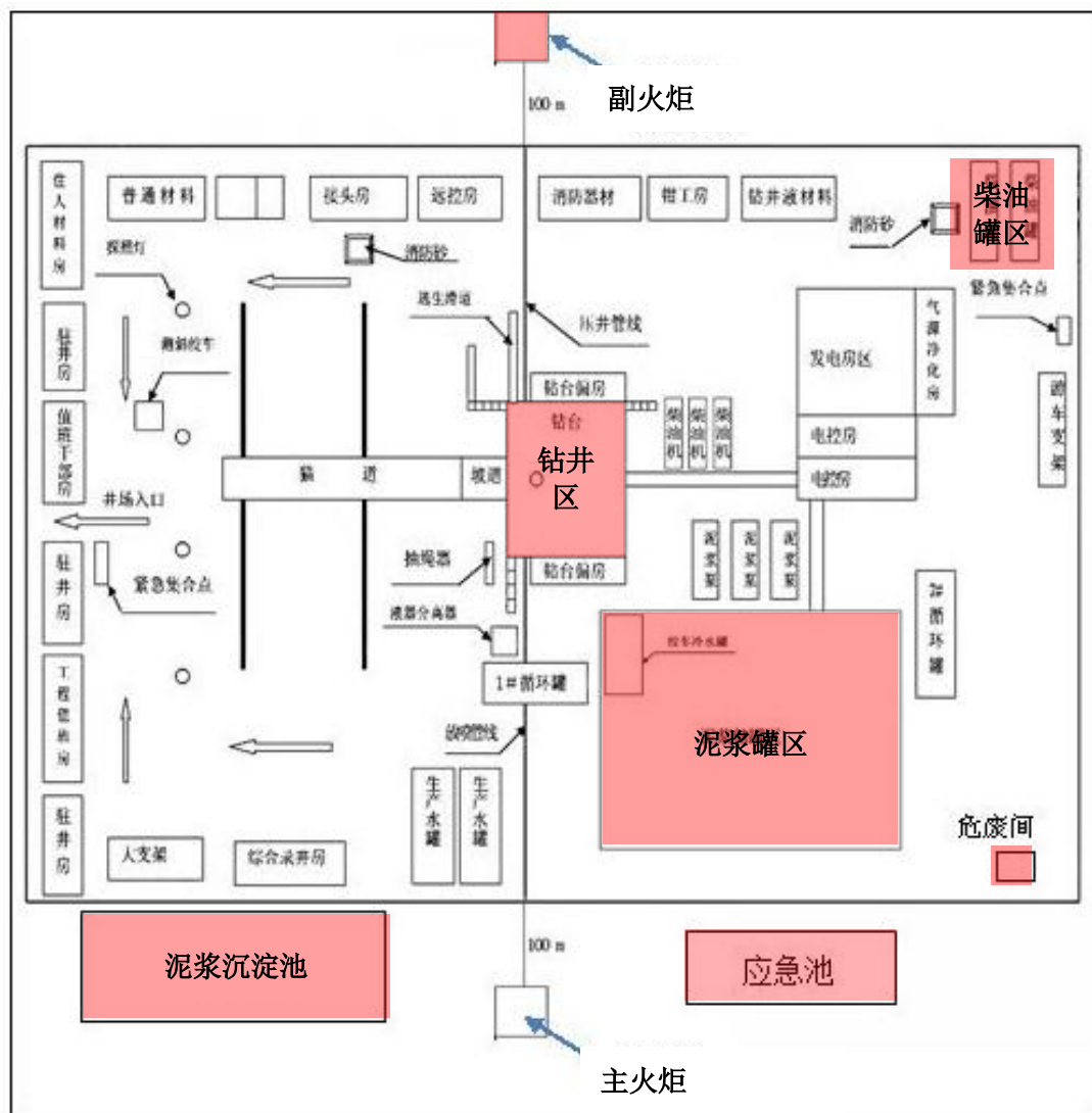
图 7 井场防渗分区图
