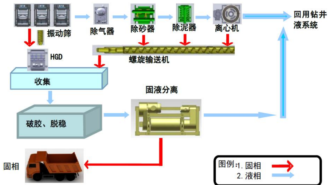
图 3 泥浆不落地系统工艺流程简图
